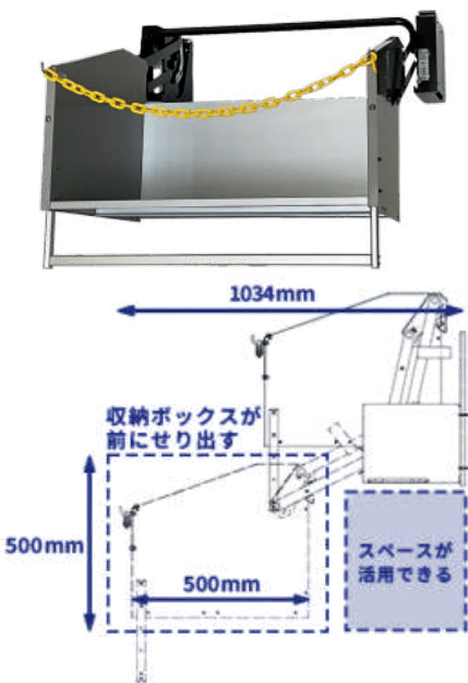
スイング式の昇降式収納棚
