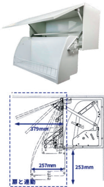
扉連動型の昇降式収納棚
