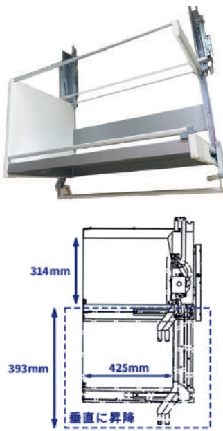
垂直式の昇降収納棚
